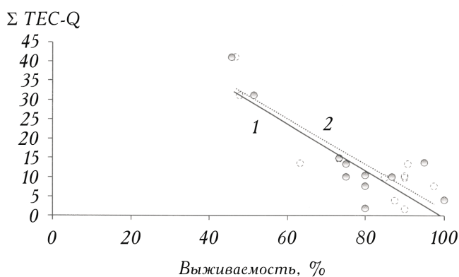
4. Связь между расчетным уровнем загрязнения донных отложений (ΣТЕС-Q) и выживаемостью тест-организмов: 1 — Daphnia magna ; 2 — Chironomus riparius .
