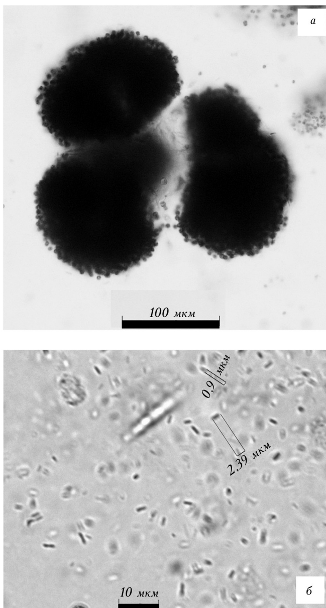
1. Внешний вид колонии Microcystis botrys (а) и фрагмент колонии Lemmermanniella flexa (б).
